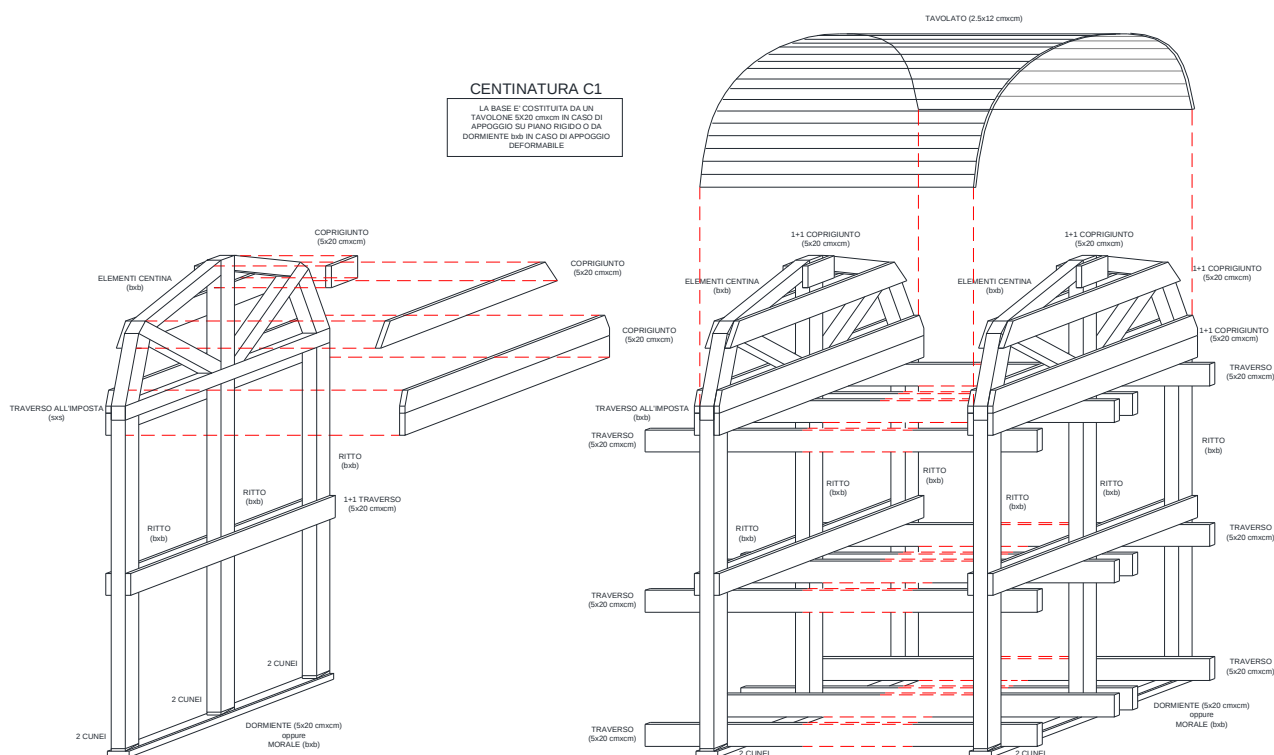
Figura 11 – Esploso assonometrico della centina lignea C1 [5]
