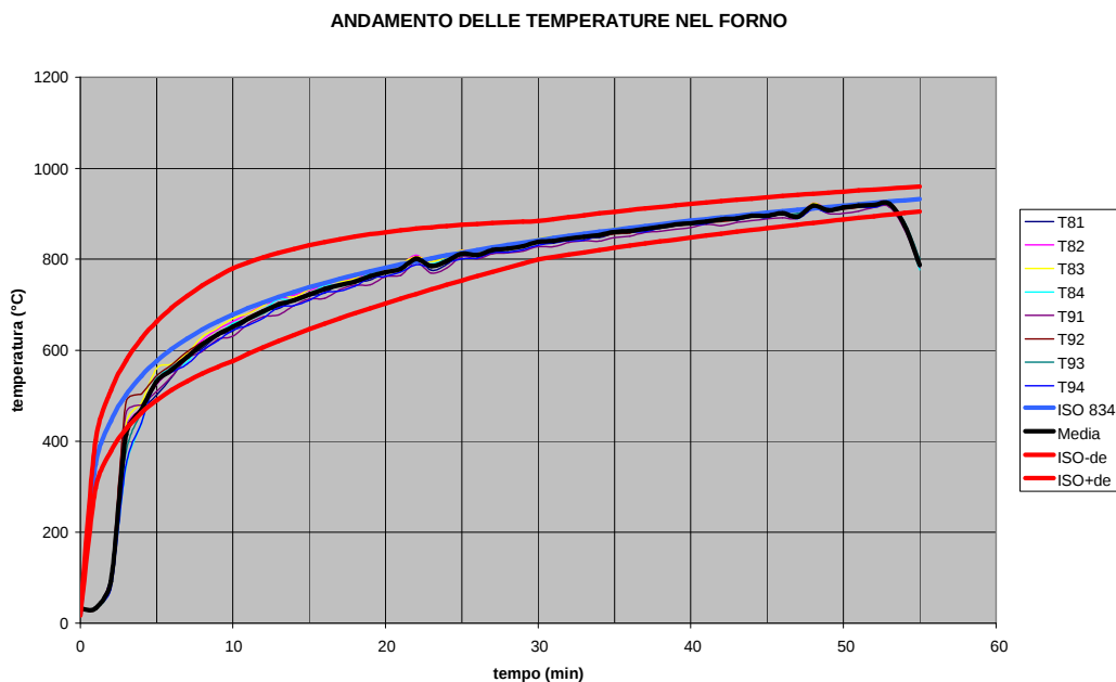
Figura 69 – Andamento delle temperature nel forno sperimentale
