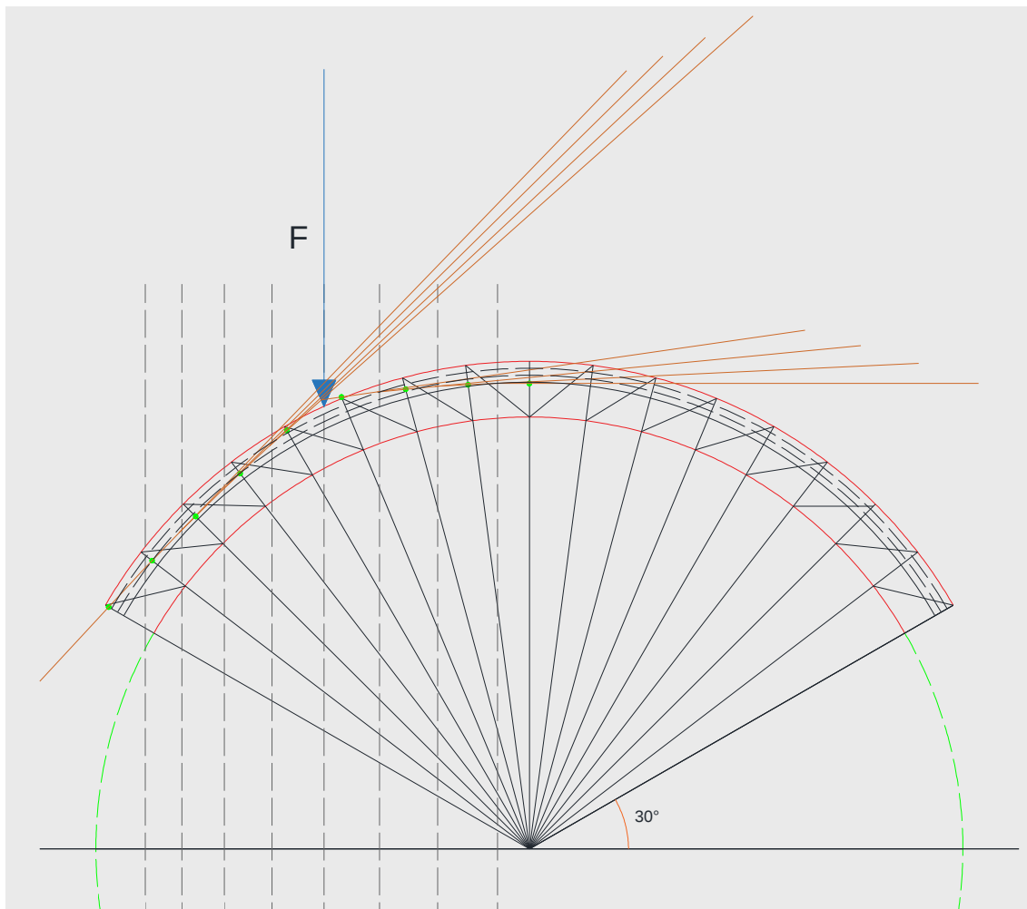
Figura 9 – Andamento del poligono funicolare dopo 60 minuti di esposizione all'incendio
