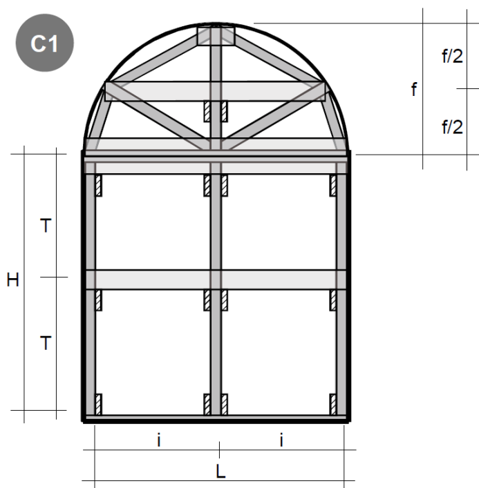
Figura 10 – Schema della centina lignea C1 [5]
