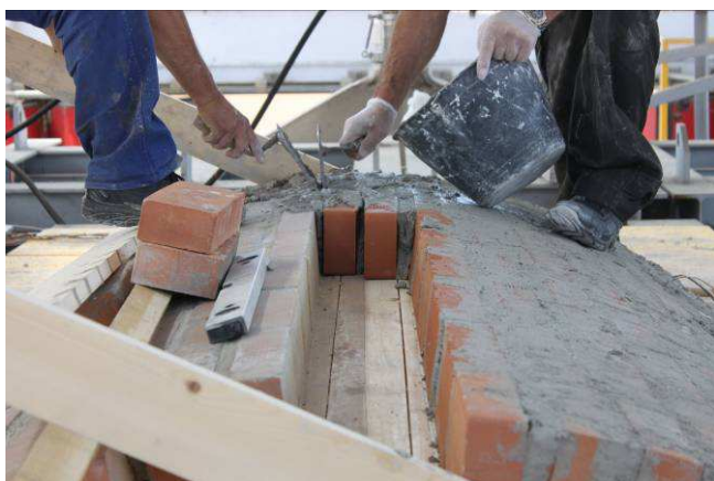
18/5/2015 – figura 36 Chiusura della chiave della volta
