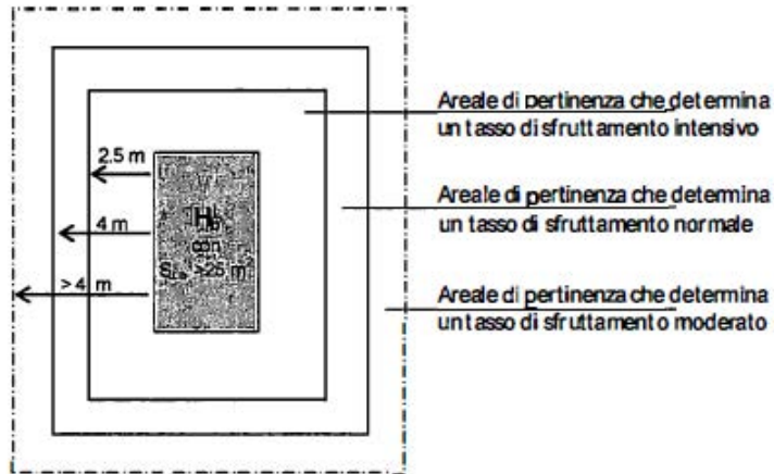
Figura 4 - Esempi di areali di pertinenza di una unità abitativa classificata H_b (con S_{a,e} > 25 \text{ m}^2 ) nel Prospetto A.3
