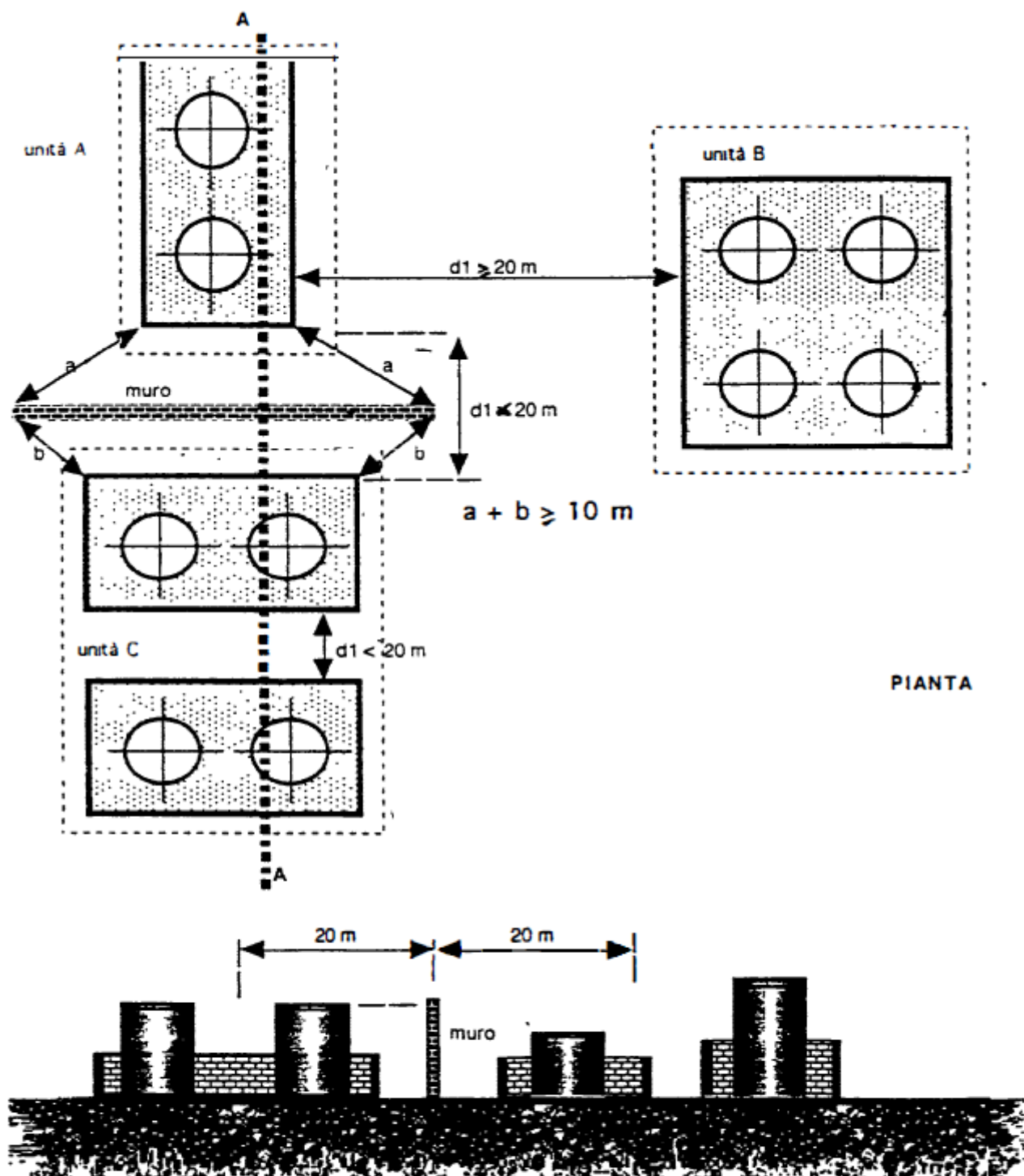
Tavola 3 - Unità di deposito all'aperto
