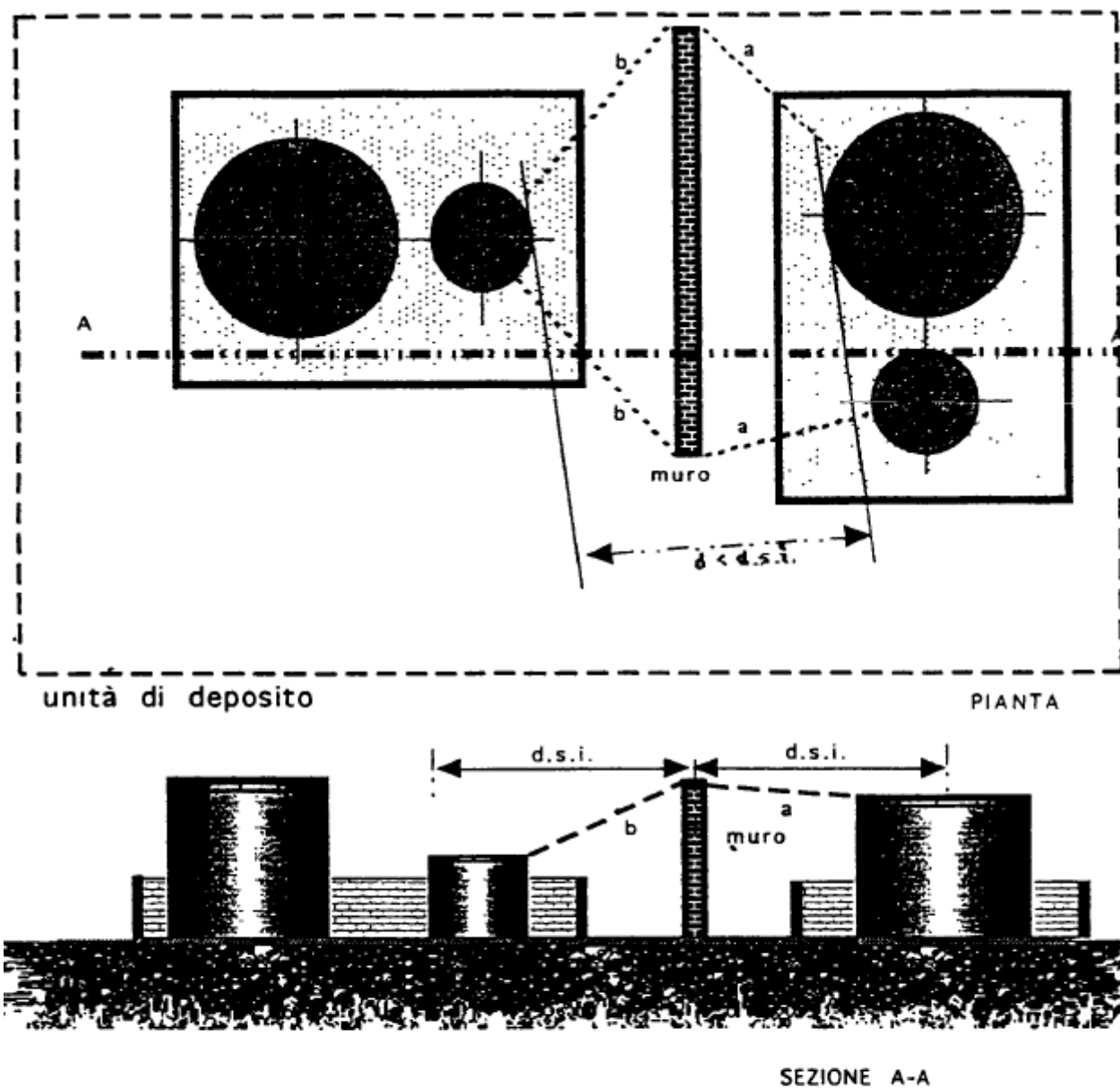
Tavola 7A - Unità di deposito all'aperto: riduzione della distanza di sicurezza interna
