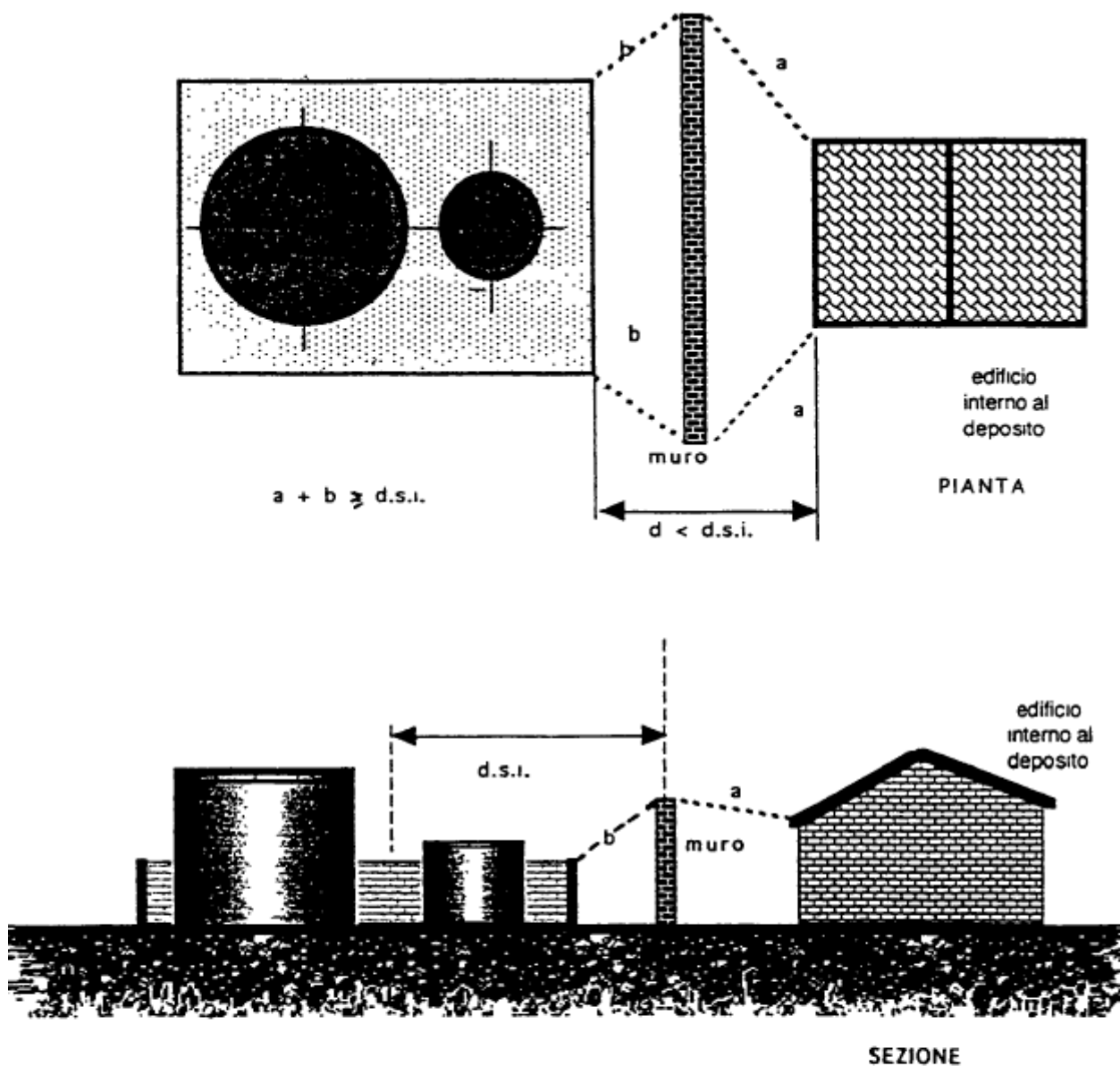
Tavola 7B - Unità di deposito all'aperto: riduzione della distanza di sicurezza interna
